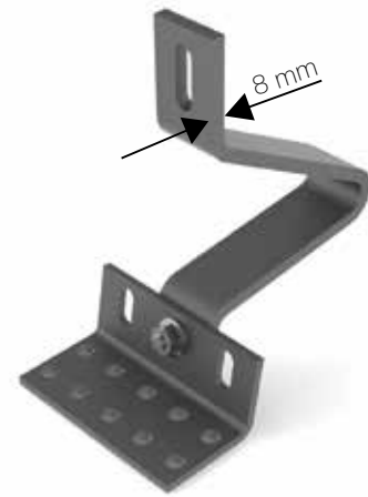
Edelstahl-Dachhaken
